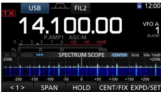
Center-Modus-Fenster
